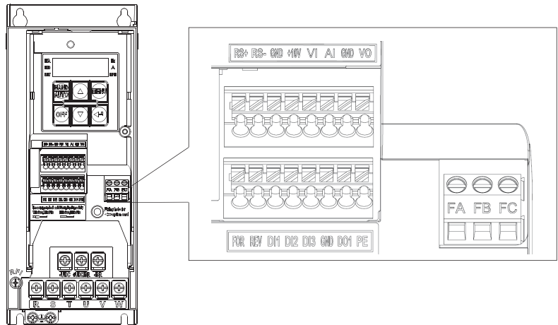
控制端子说明：
