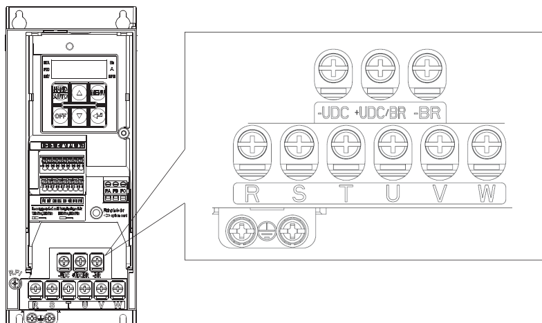
主回路端子示意图
