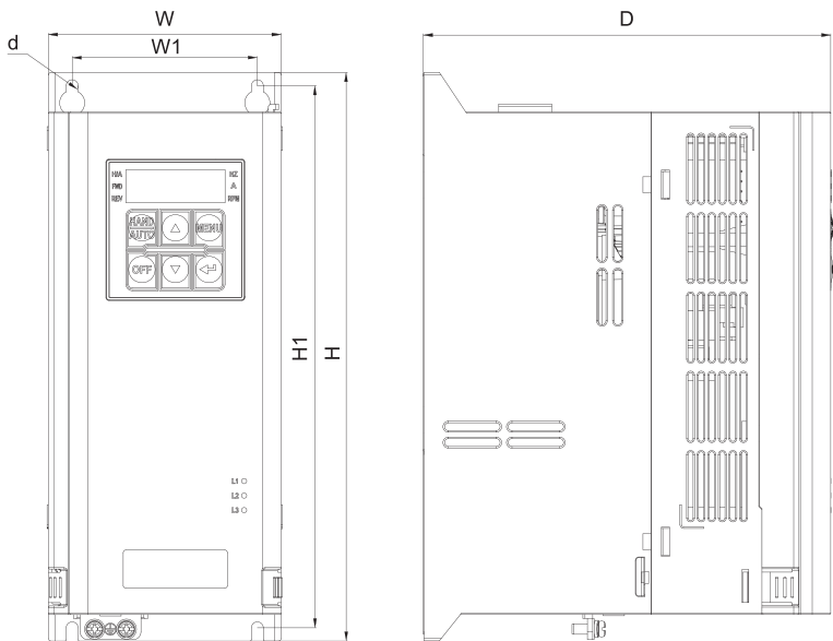
NA0-B~NA2 机箱
