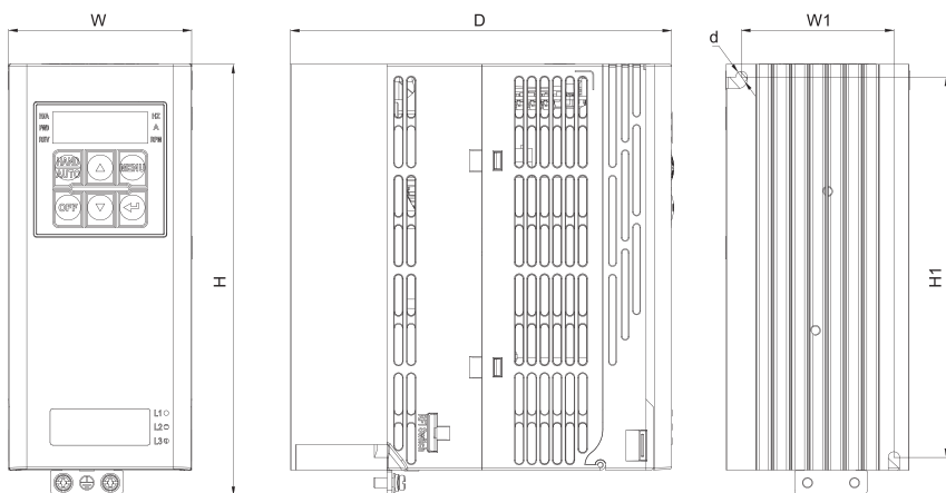
NA0-A 机箱
