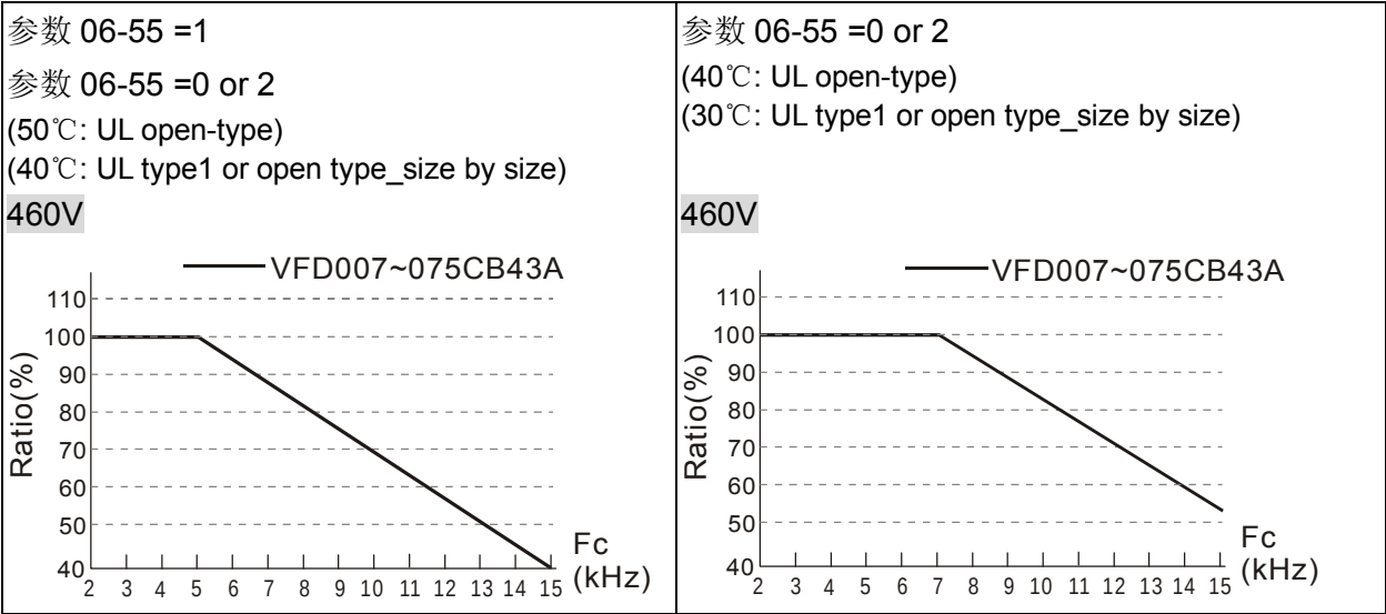
Heavy Duty 之降载曲线图 (参数 00-16=1)
