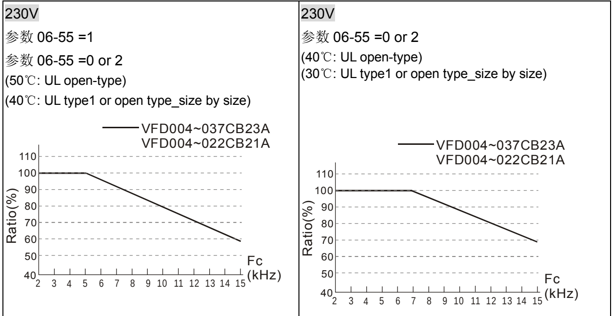
Normal Duty 之降载曲线图(参数 00-16=0)
