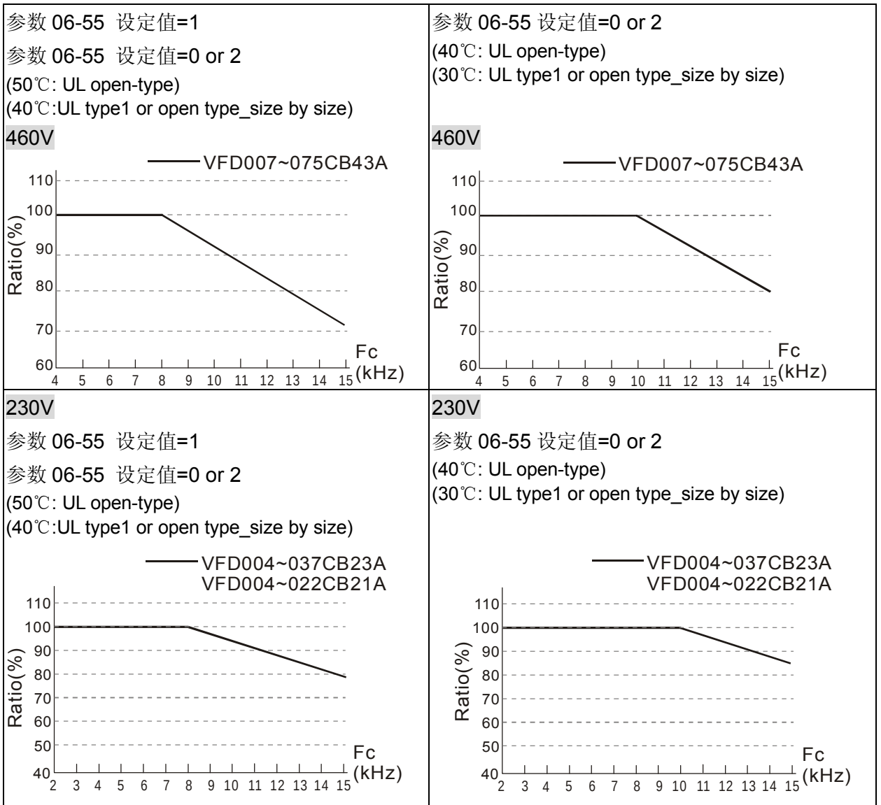
Normal Duty 之降载曲线图(参数 00-16=0)
